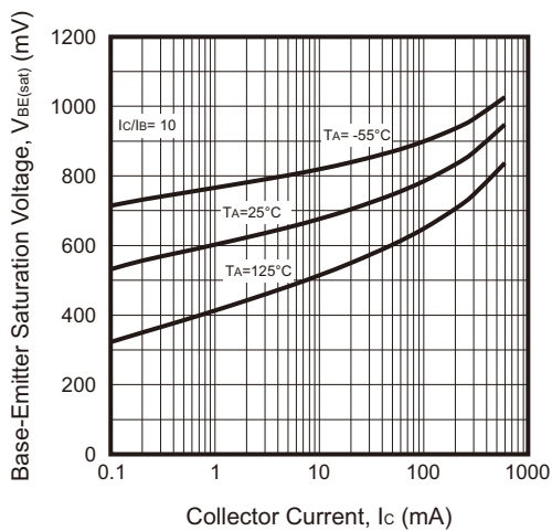
Fig.3 - V_{BE(sat)} - I_c
