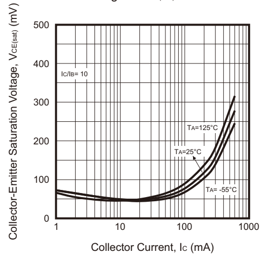
Fig.2 - V_{CE(sat)} - I_c
